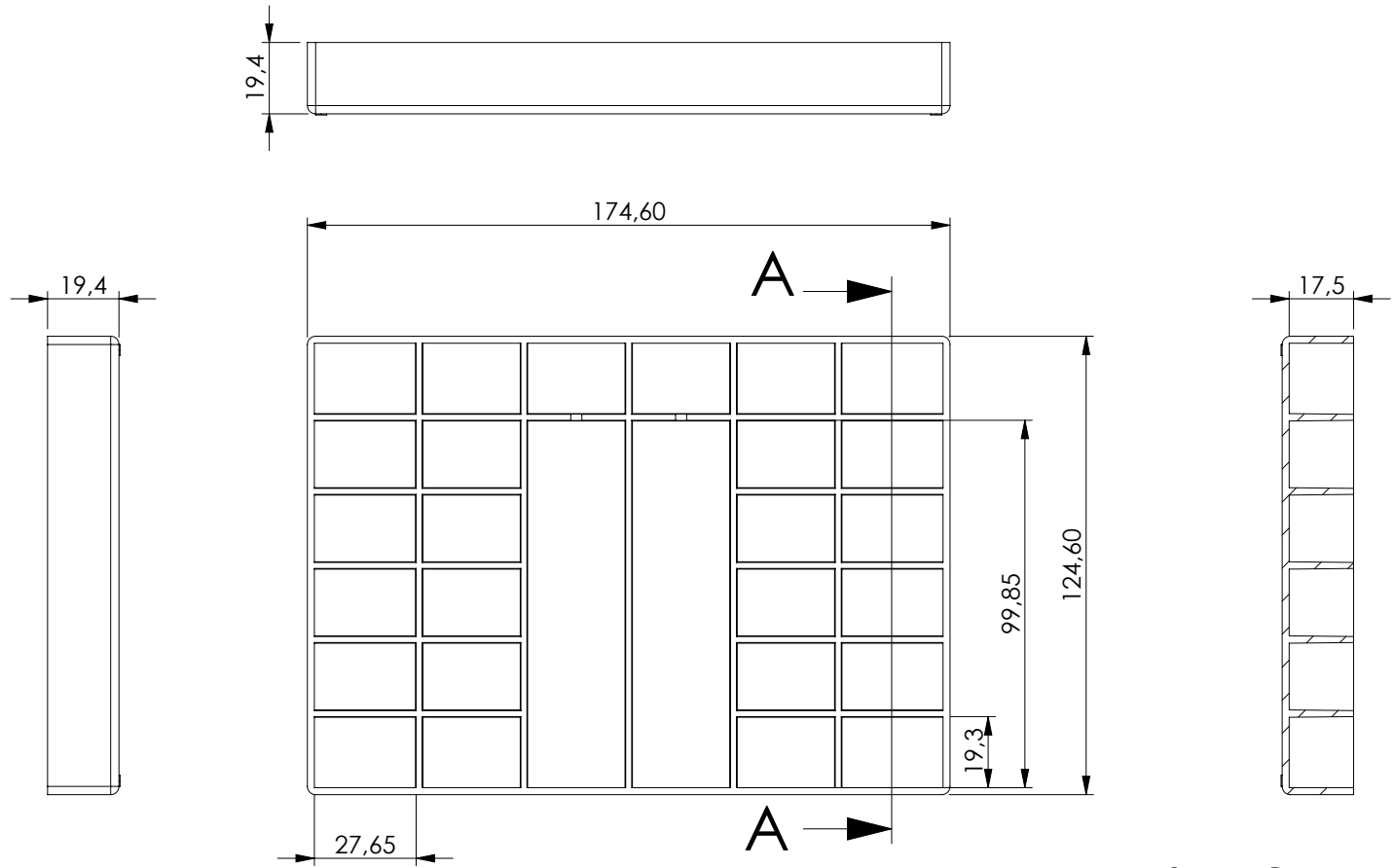
SEZIONE A-A
